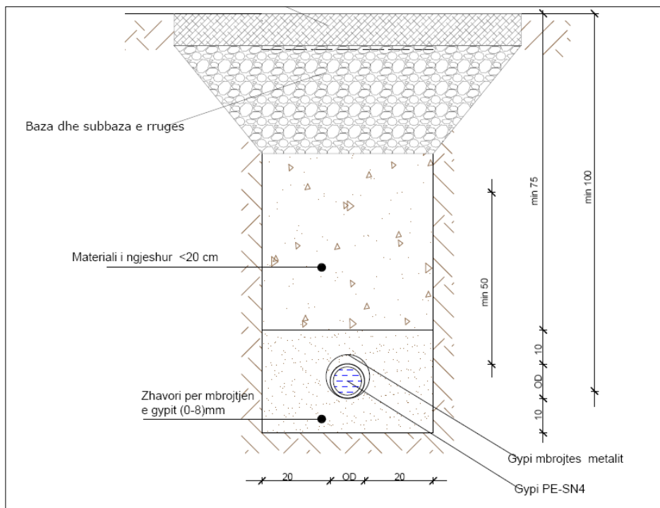
Fig. 16: Prerja karakteristike për kanalin e kanalizimit
