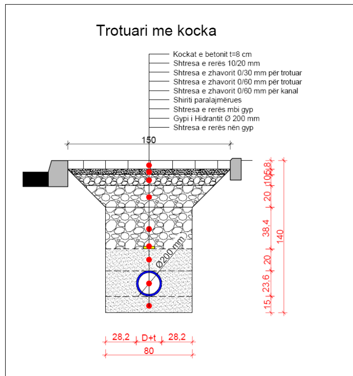
Fig. 15: Prerja karakteristike për kanalin e ujësjetës
